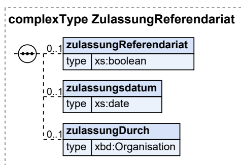
Abbildung II.1.6. ZulassungReferendariat
