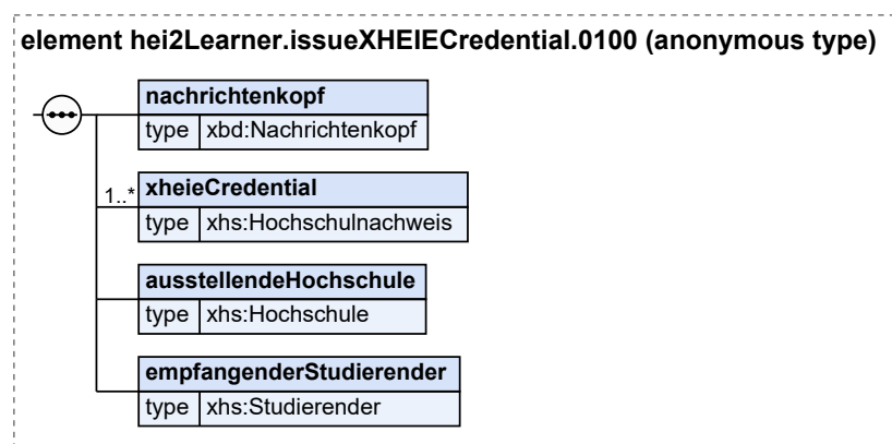
Abbildung III.1.1. hei2Lerner.issueXHEIECredential.0100
