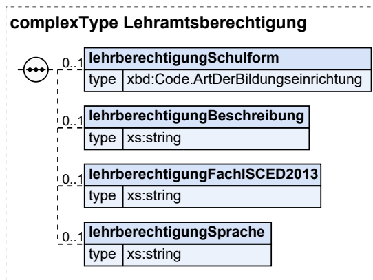
Abbildung II.1.3. Lehramtsberechtigung
